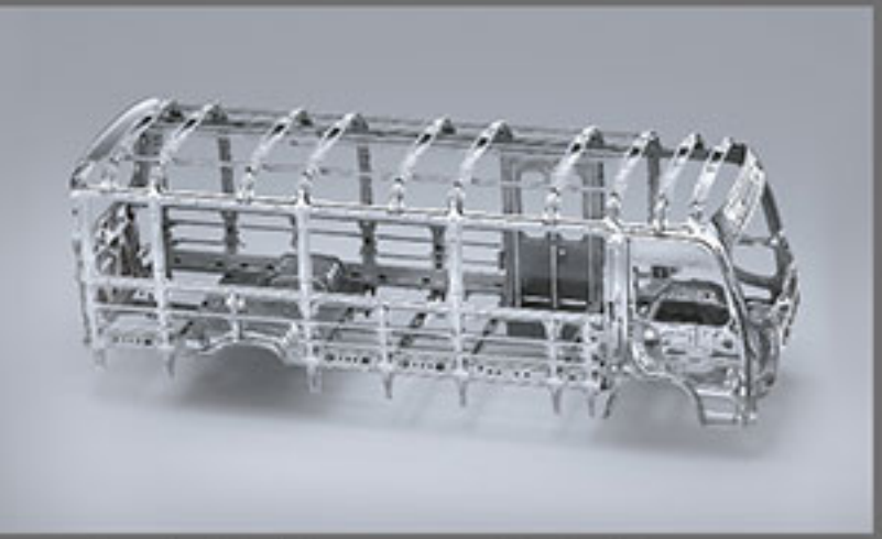
โครงสร้างตัวถังพร้อมคานเสริมนิรภัย พัฒนาออกแบบอย่างเป็นพิเศษ ให้แข็งแรงยิ่งขึ้น กระจายแรงกระแทกเพื่อปกป้องผู้โดยสาร จากการชนได้อย่างดีเยี่ยม
