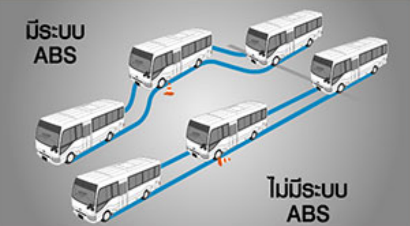
ระบบเบรก ABS (Anti-lock Braking System) ป้องกันล้อล็อกและลื่นไถลทำให้สามารถควบคุมรถ และหลบเลี่ยงสิ่งกีดขวางได้ เมื่อรถเบรกกระทันหัน
